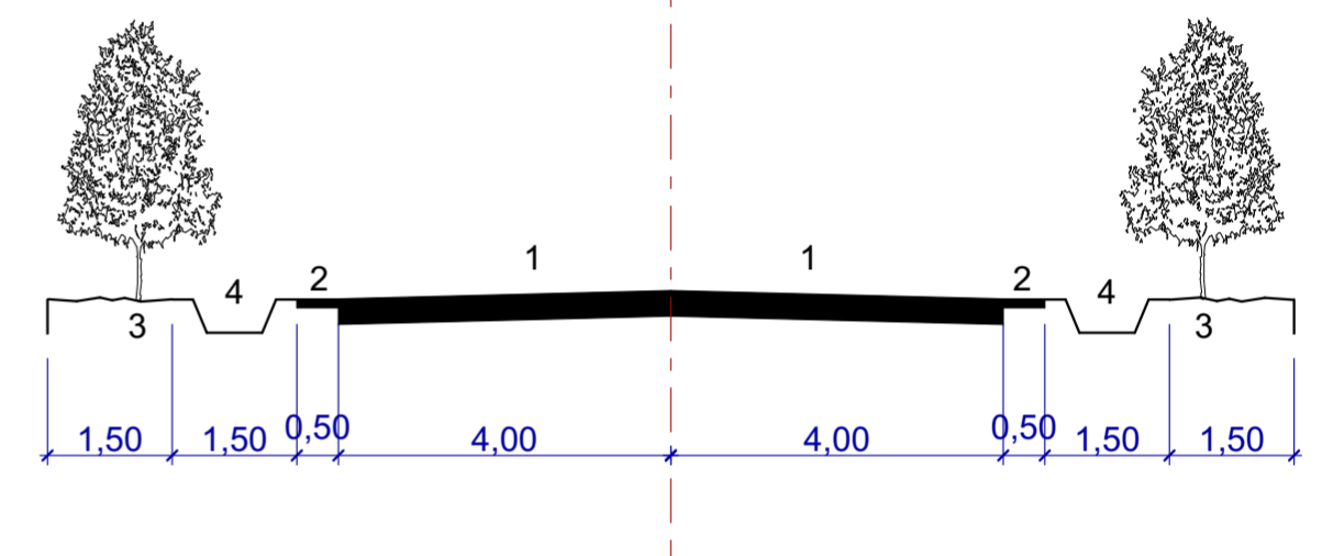
1. Поперечний профіль дороги
